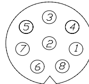
Stiftgehäuse 7-polig Ansicht A
