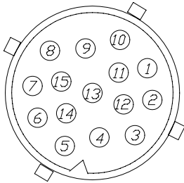
Stiftgehäuse 15-polig Ansicht A
