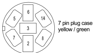
Kupplung 7-pol. gelb und grün
